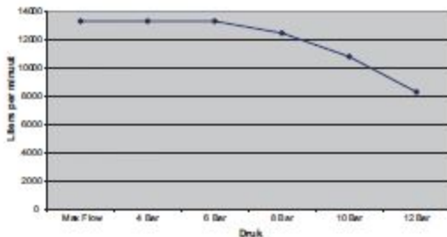
Capaciteitscurve
